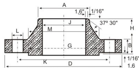
Figura 1115 - FLANGE COM PESCOÇO
