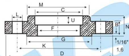
Figura 1315 - FLANGE DE ENCAIXE
