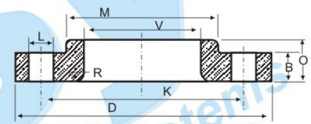
Figura 1515 - FLANGE SOLTO
