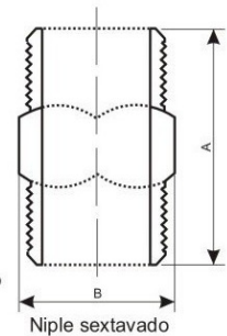
Figura 2931 - Niple para alta pressão - 3000 IBS - Neg 1 corpo Figura 2810 - Niple Sextavado em Aço Rosca BSP Figura 2820 - Niple Sextavado em Aço Rosca NPT Figura 2830 - Niple Sextavado em Aço Carbono BSP Figura 2840 - Niple Sextavado em Aço Carbono NPT
